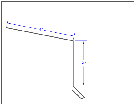
58 Dekk - Tile Eave 6"
