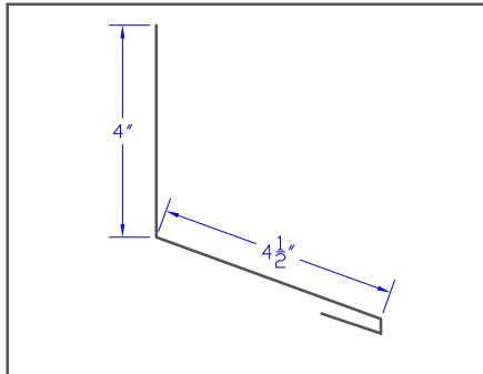
59 Dekk - Tile End Wall 9"
