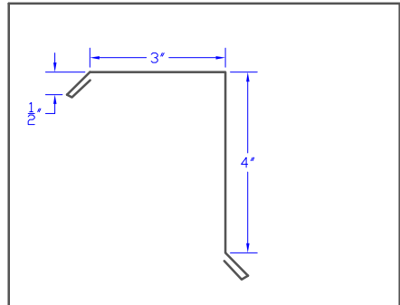
57 Dekk - Tile Gable Trim 9"
